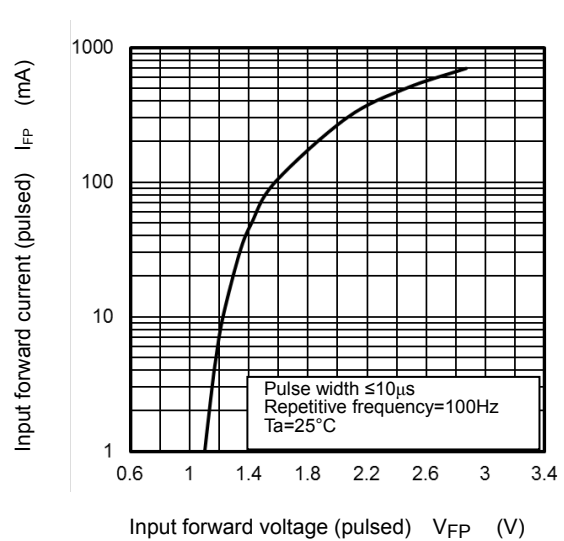
I_{FP} - V_{FP}
