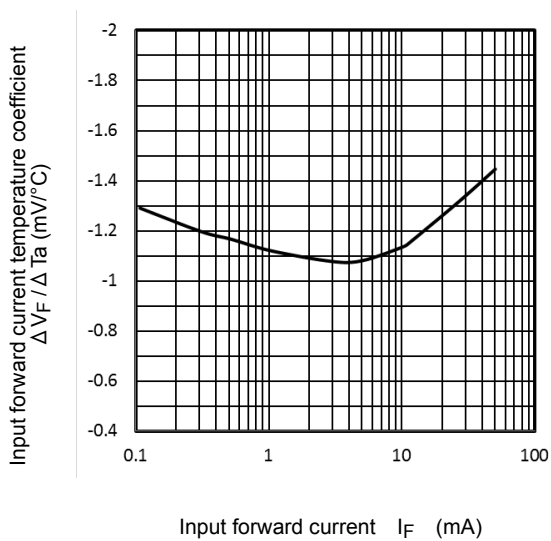
\Delta V_F / \Delta T_a - I_F
