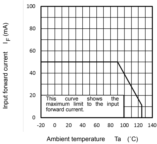
I_F - T_a
