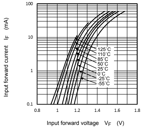
I_F - V_F
