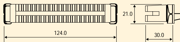
10 Pair Module
