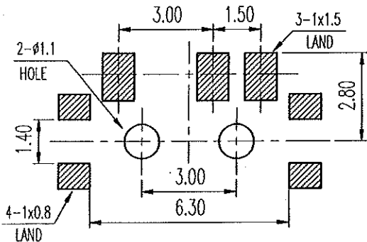
安装孔 PIERCING PLAN
