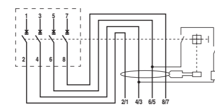
DDA 804
