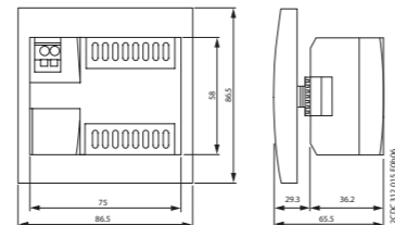
CL-LDC.S..
