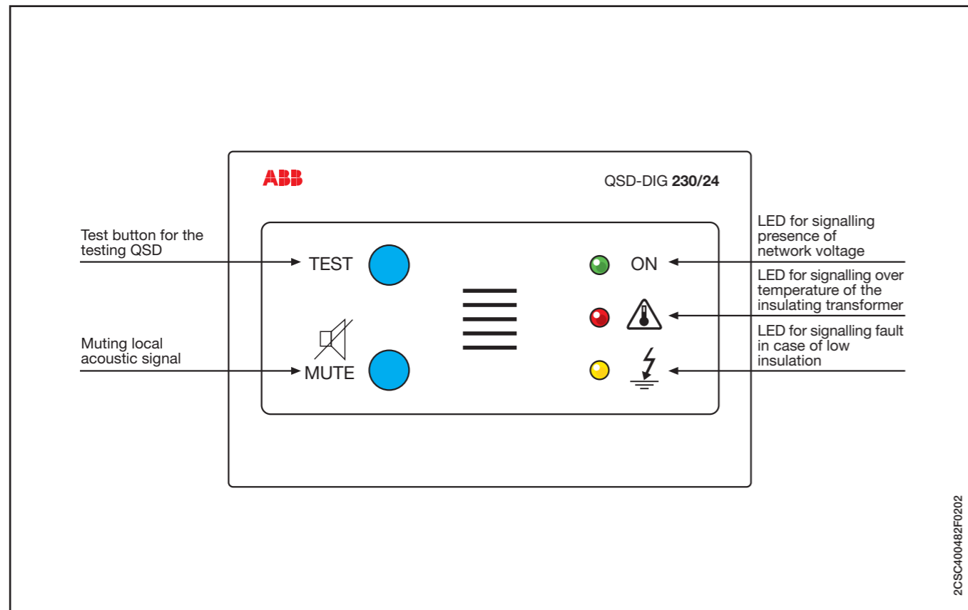
QSD-DIG 230/24
