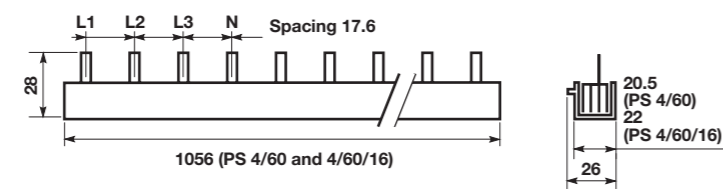
PS 4/60
