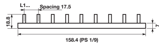
PS 1/9
