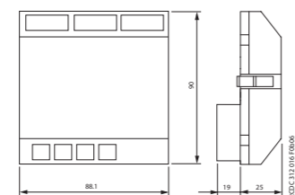
CL-LDR, CL-LDT
