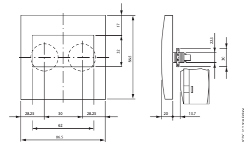
CL-LDD
