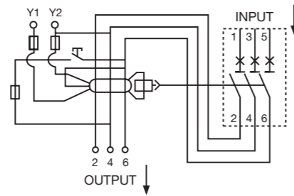
DDA 203 AE
