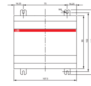
CL-LMR, CL-LMT
