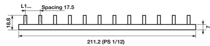
PS 1/12
