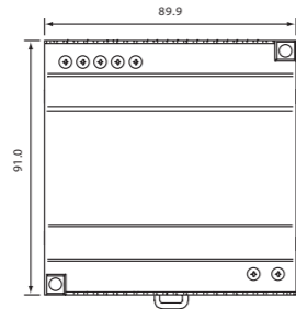
CP-D 24/4.2
