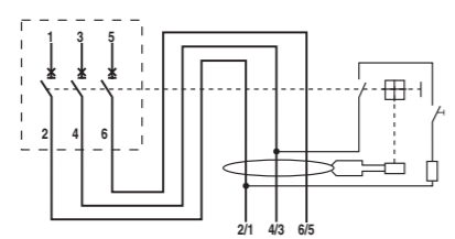
DDA 803
