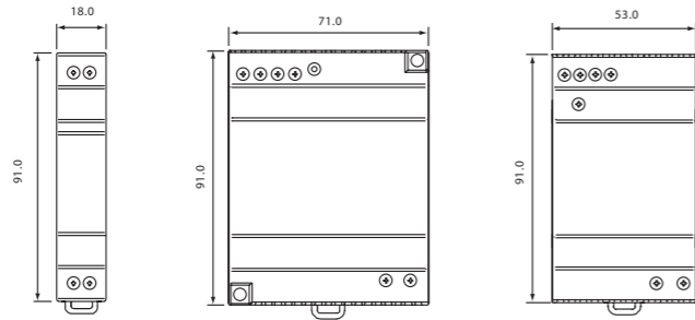
CP-D 12/0.83, CP-D 24/0.42
