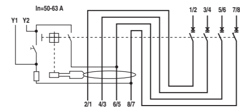
DS 204
