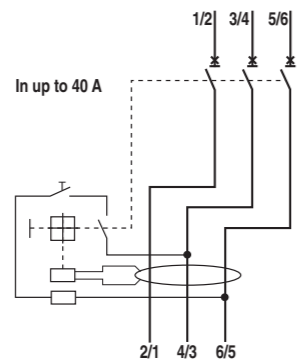
DS 203
