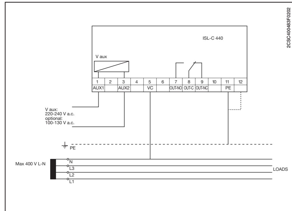
ISL-C 440
