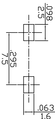
P.C.B. LAND DIMENSION
