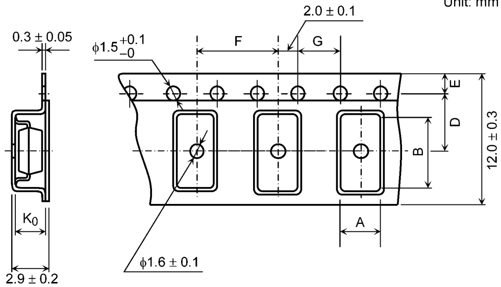
Fig. 16.3.5.1 Tape dimensions
