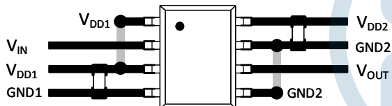
图 9.推荐的印刷电路板布局
