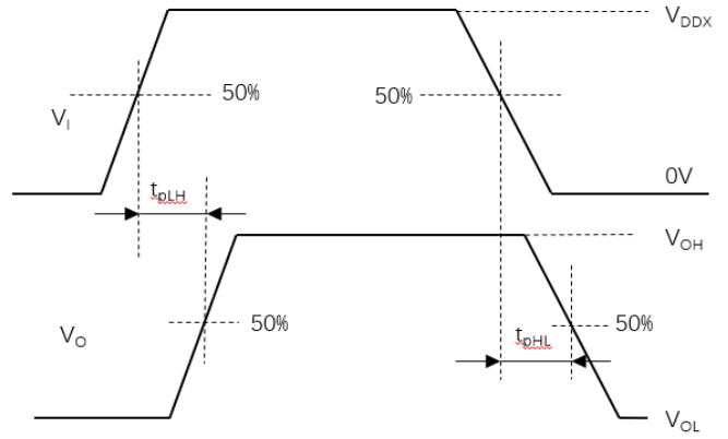
图 8.传输延迟时间波形测量
