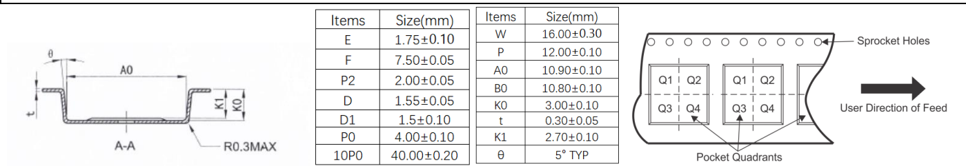
图 28.16 引脚宽体 SOIC 封装 [WB SOIC-16] 包装信息
