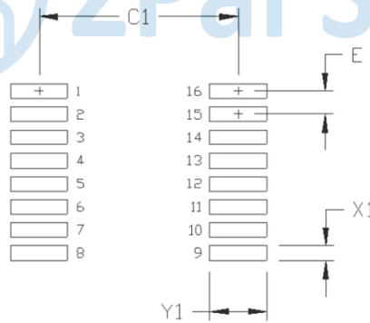
图 24. 16 引脚 SSOP 封装 [16-Lead SSOP] 焊盘图案
