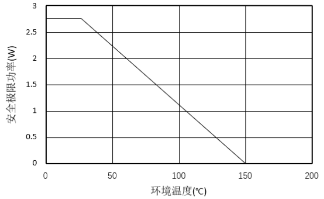
图 6.热降额曲线，依据 DIN V VDE V 0884-10 的安全限值与环境温度的关系(左: π14xM3x; 右: π14xM6x)
