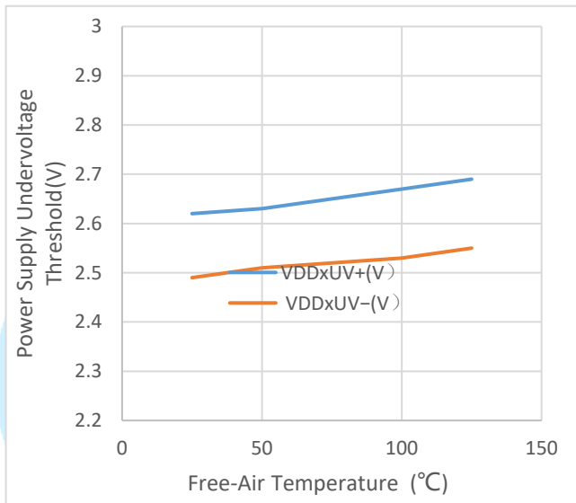
图 7.UVLO vs. 空气温度
