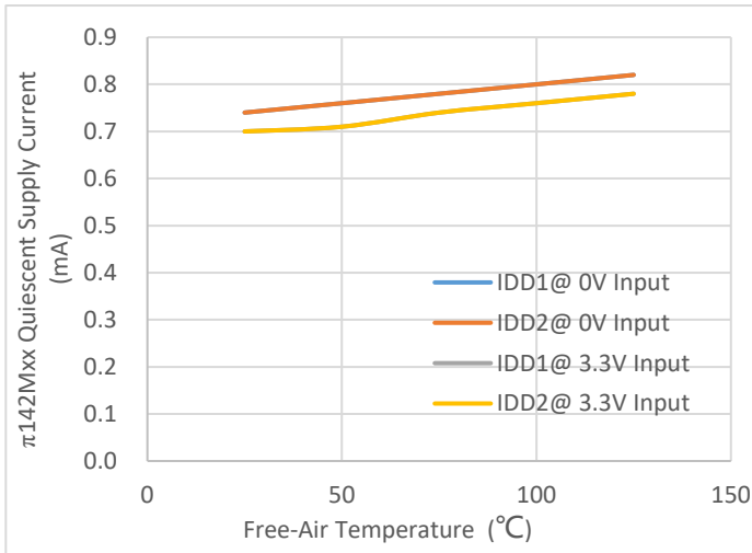
图 13. 3.3V 供电, \pi 142Mxx 静态供电电流 vs. 空气温度
