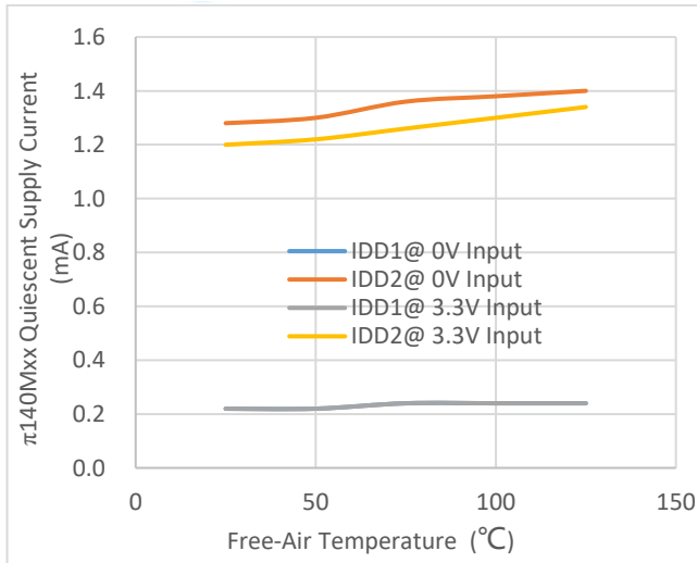
图 9. 3.3V 供电，π140Mxx 静态供电电流 vs. 空气温度
