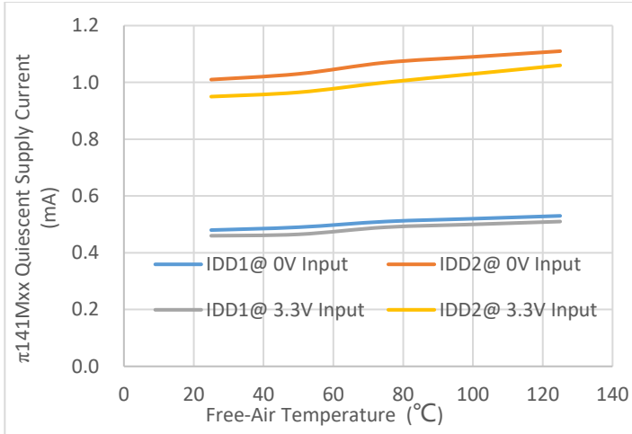
图 11. 3.3V 供电, \pi 141Mxx 静态供电电流 vs. 空气温度
