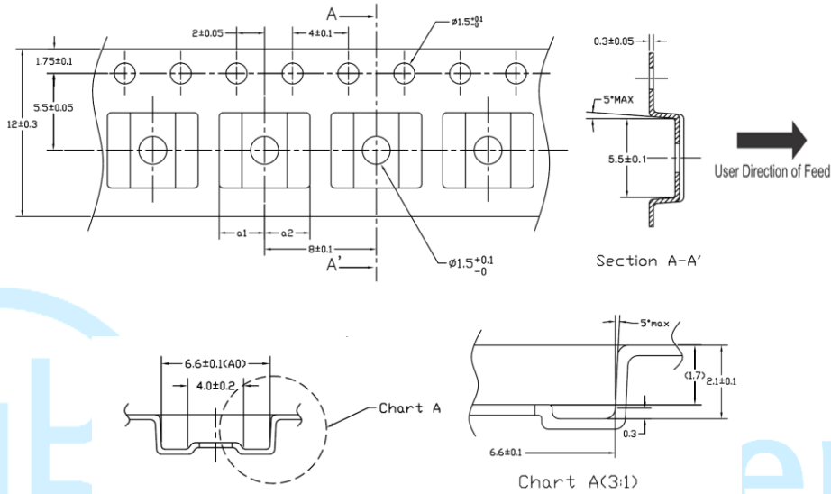
图 29.16 引脚宽体 SSOP 封装包装信息
