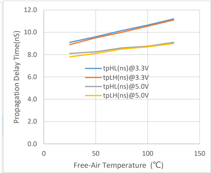
图 8.传输延时 vs. 空气温度
