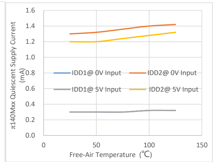
图 10. 5V 供电，π140Mxx 静态供电电流 vs. 空气温度
