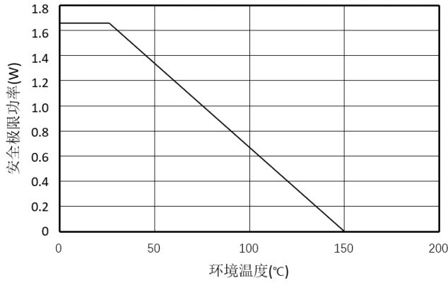
图 6.热降额曲线，依据 DIN V VDE V 0884-10 的安全限值与环境温度的关系(左: π14xM3x; 右: π14xM6x)
