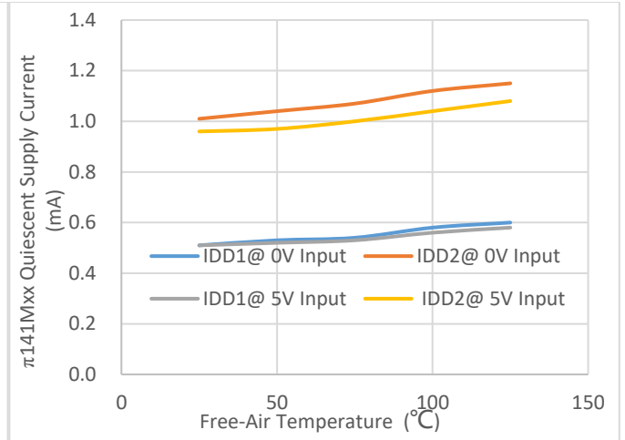
图 12. 5V 供电, \pi 141Mxx 静态供电电流 vs. 空气温度
