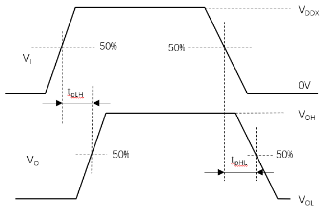
图 16. 传输延迟时间波形测量
