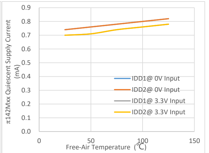
图 14. 5V 供电, \pi 142Mxx 静态供电电流 vs. 空气温度
