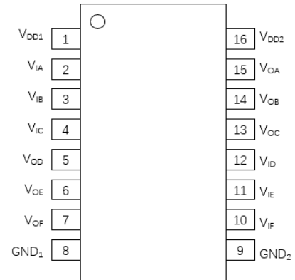
图 6. \pi 163Uxx 管脚定义
