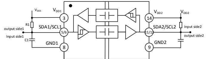
图 20. \pi 220N61 系统工作图
