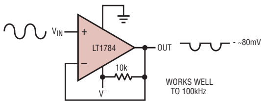
Negative Rectifier
