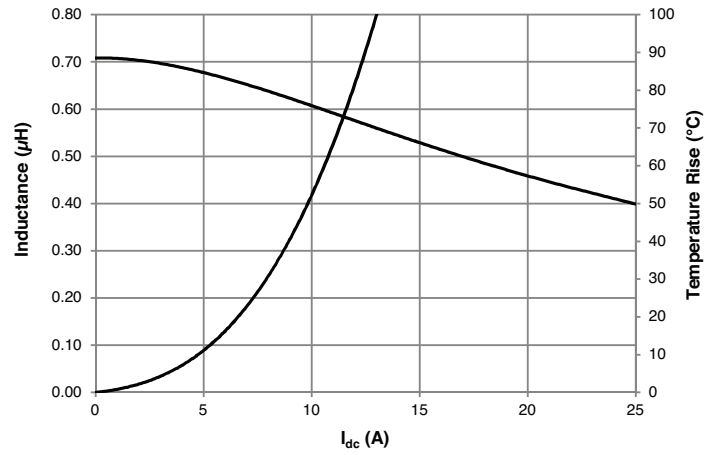
HCM1A0503-R75-R
