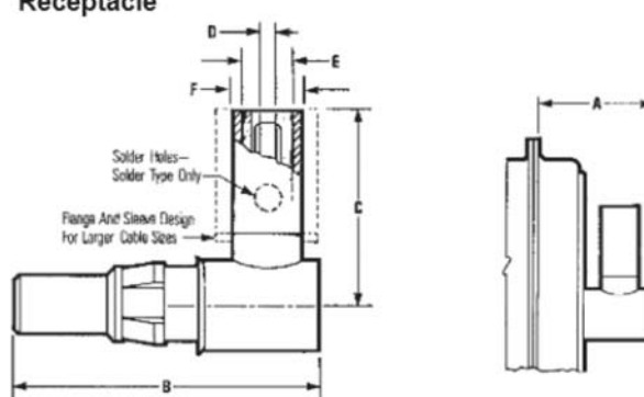
Receptacle
