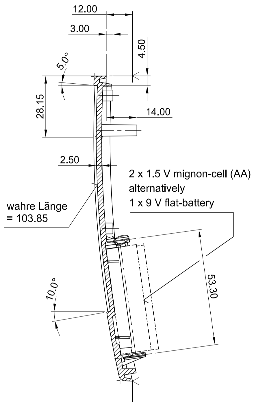
Schnitt B-B section
