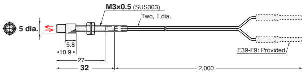
19-C E32-C31 2M (Free Cutting) + E39-F3C
