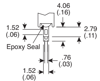
SOLDER LUG
