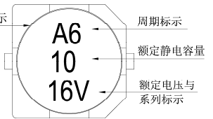
负极标示
