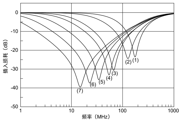
SA型 (AC400V(r.m.s.))
