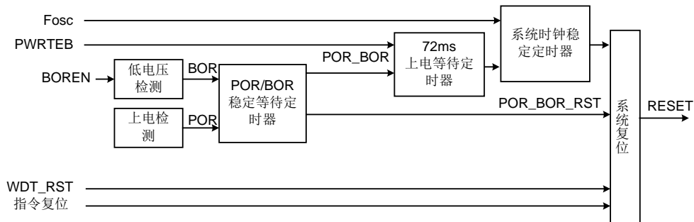
图 6-8 芯片复位原理图
