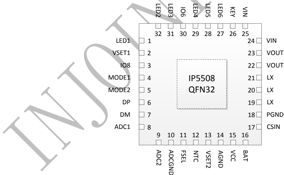
图 2 IP5508 引脚图
