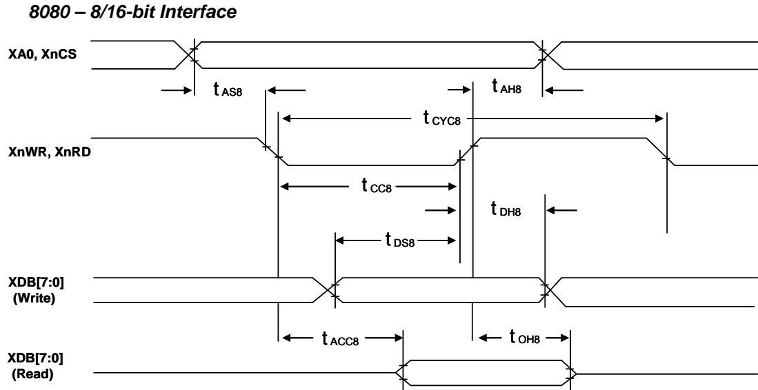
圖 7-3 : 8080 Waveform
