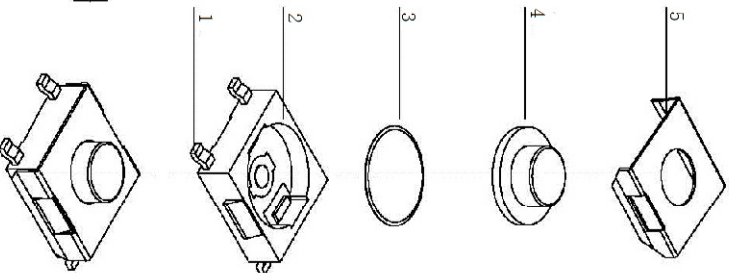
3D轴测图
