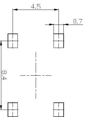
安装参考图
