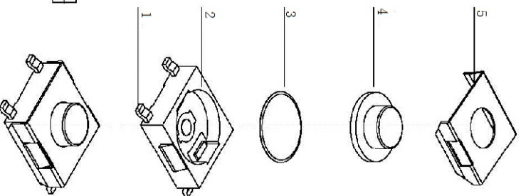
3D轴测图
