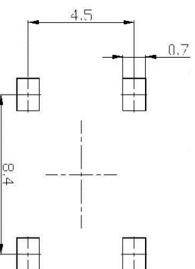
安装参考图
