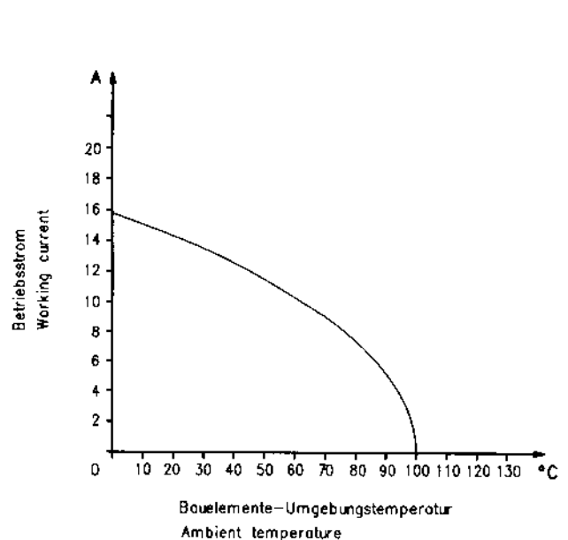
Anschlußquerschnitt 1,5 mm 2 wire gauge 1,5 mm 2
