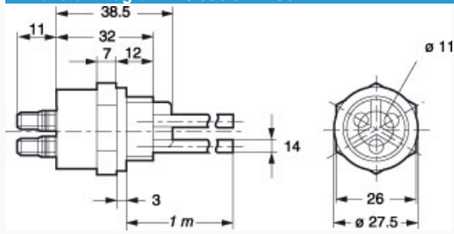
Dimension Diagram : 79 696 044 - S8
