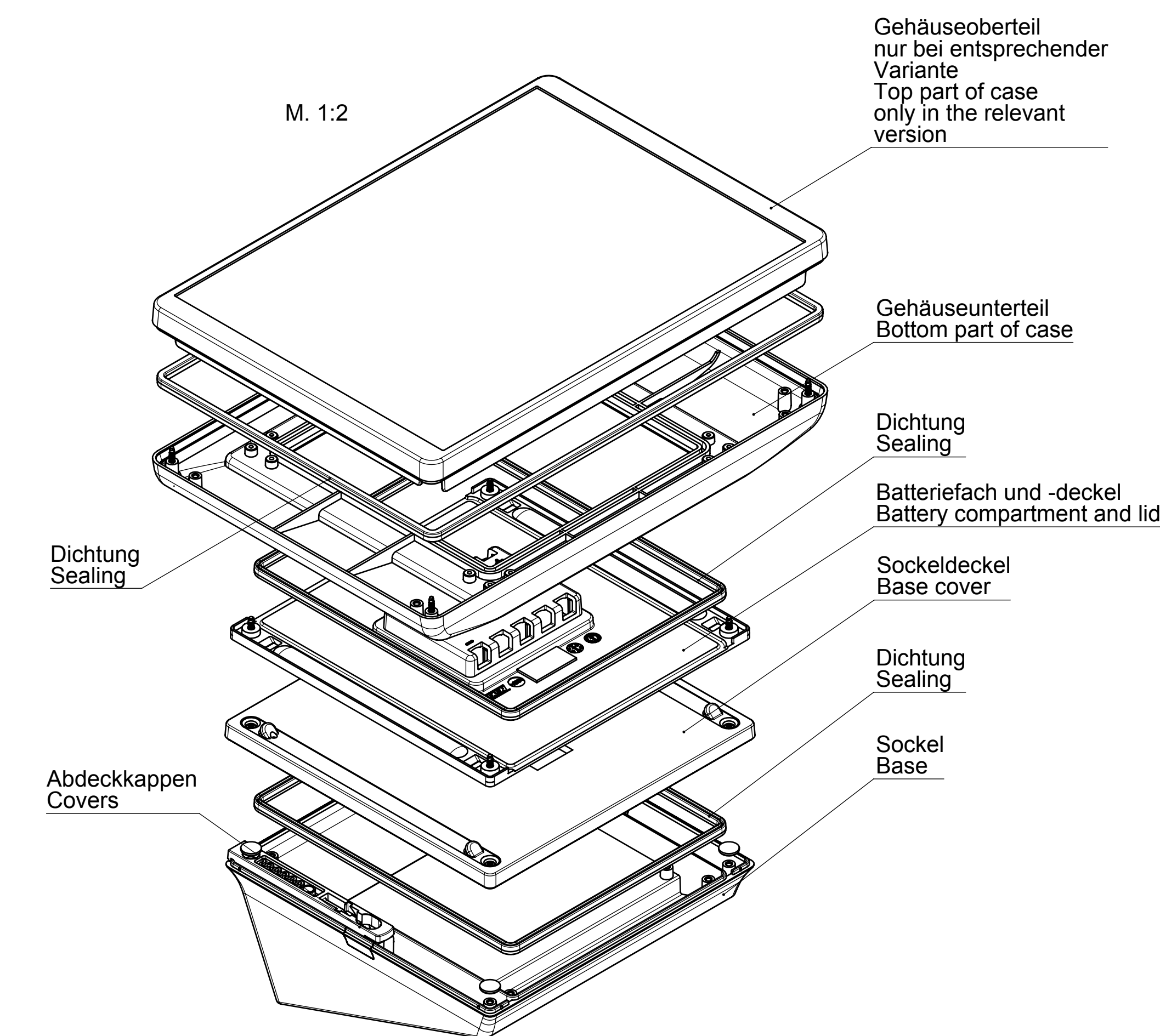
B 40 46 167 mit Gehäuseoberteil with top part
