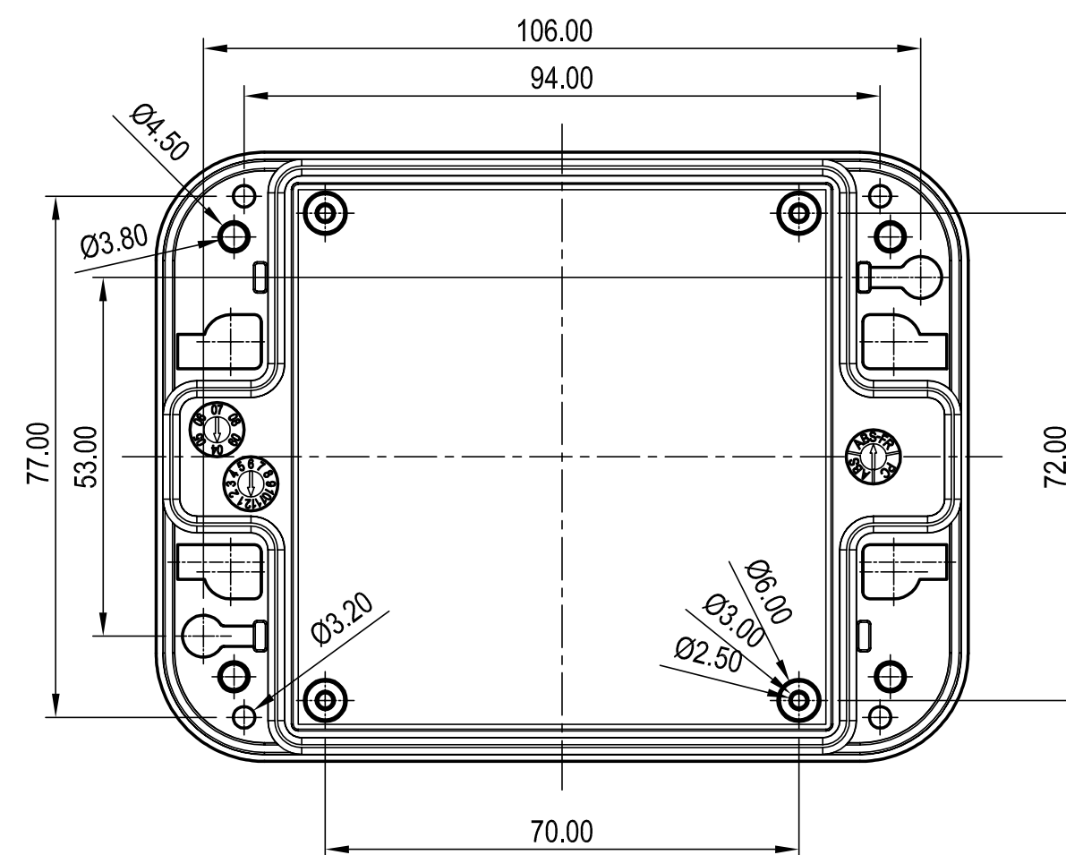
Oberteil Innenansicht Top part inside view
