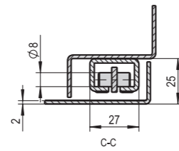
Verschlusshalter Catch
