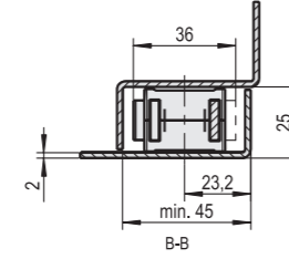
Stangenschloss Locking bolt
