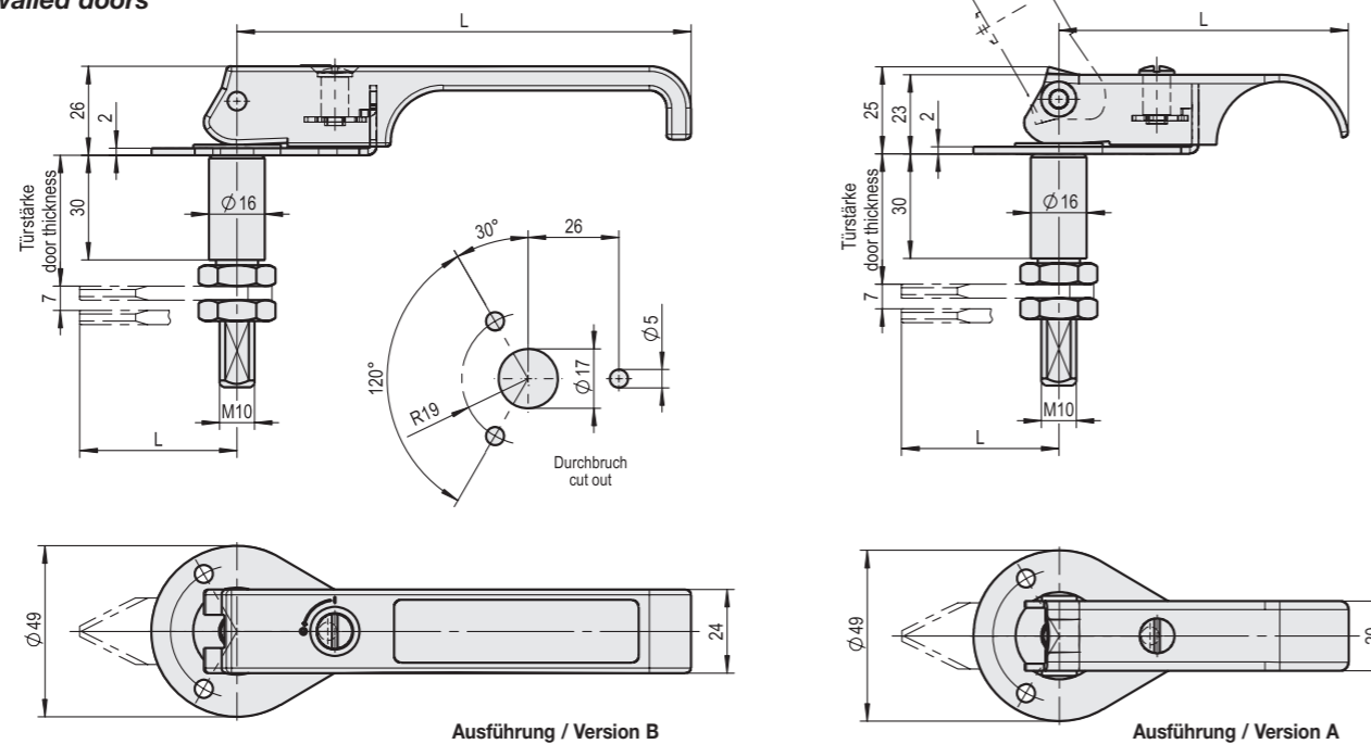
Ausführung / Version B
