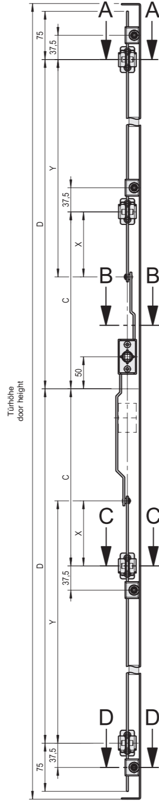
Verschlusshalter Catch
