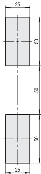
Durchbruch cut out
