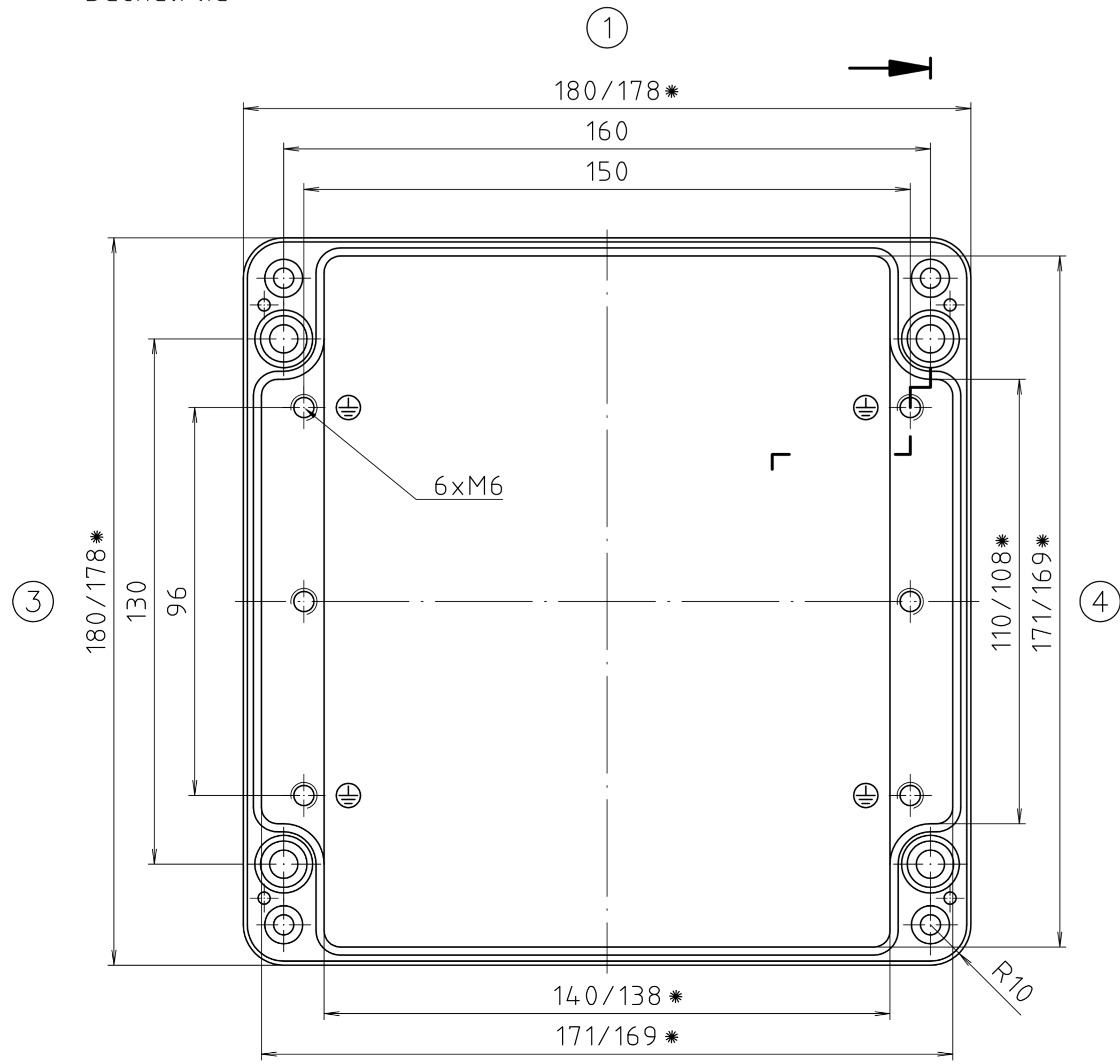
Unterteil/base
