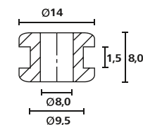
HV1208
