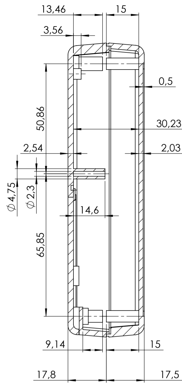
SEZIONE A-A
