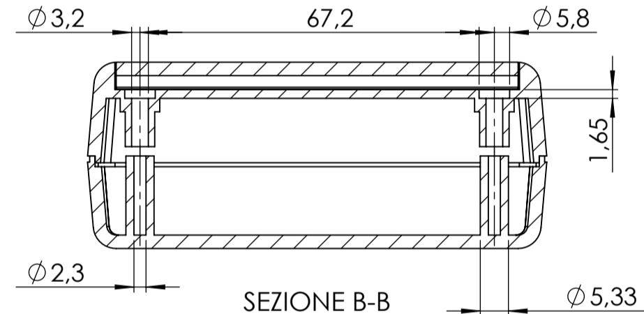
SEZIONE B-B
