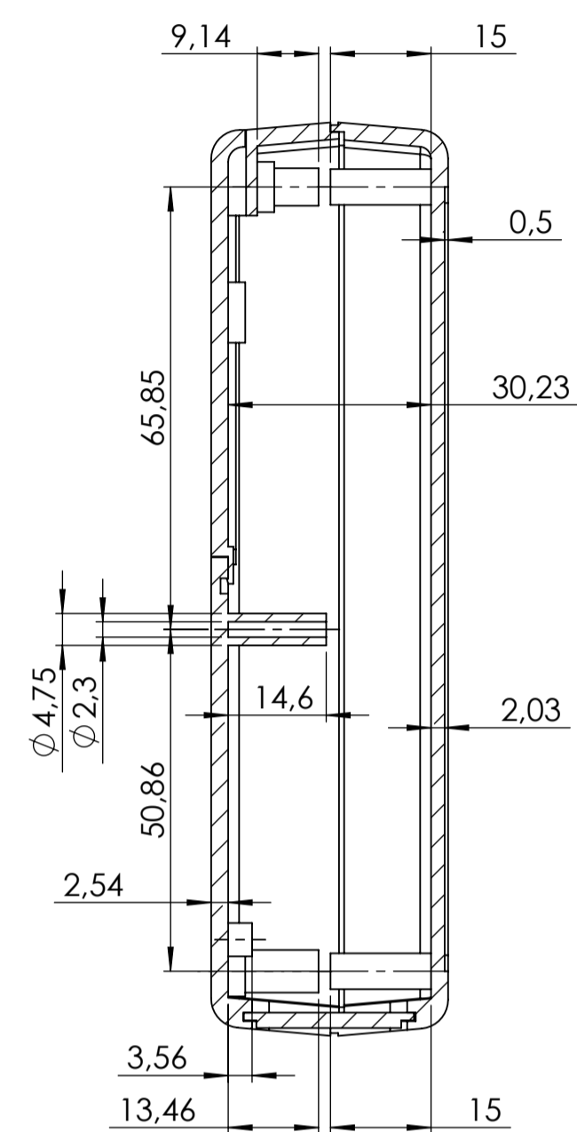
SEZIONE A-A
