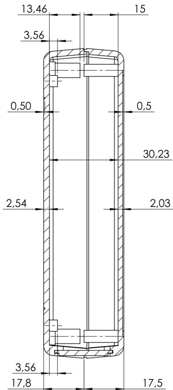
SEZIONE A-A
