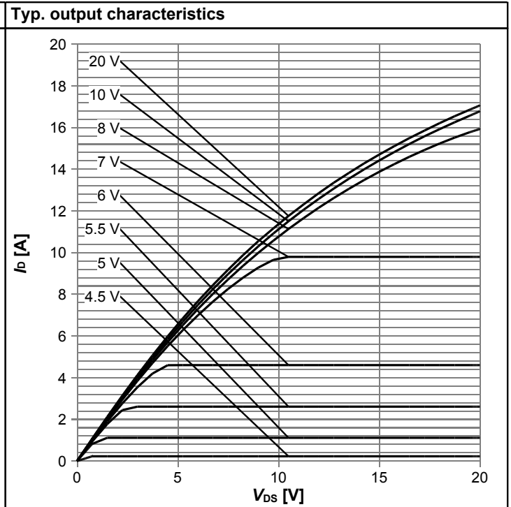
I_D=f(V_{DS}); T_j=125\text{ °C}; \text{parameter: } V_{GS}
