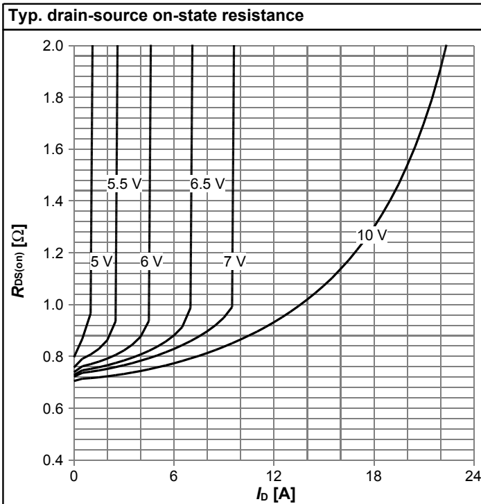
R_{DS(on)}=f(I_D); T_j=125\text{ °C}; \text{parameter: } V_{GS}
