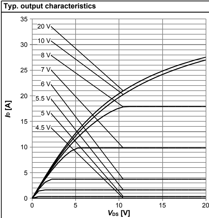
I_D=f(V_{DS}); T_j=25\text{ °C}; \text{parameter: } V_{GS}
