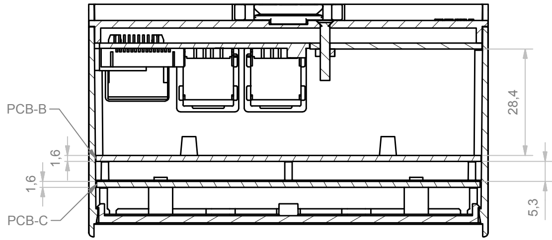
A-A (1:1)
