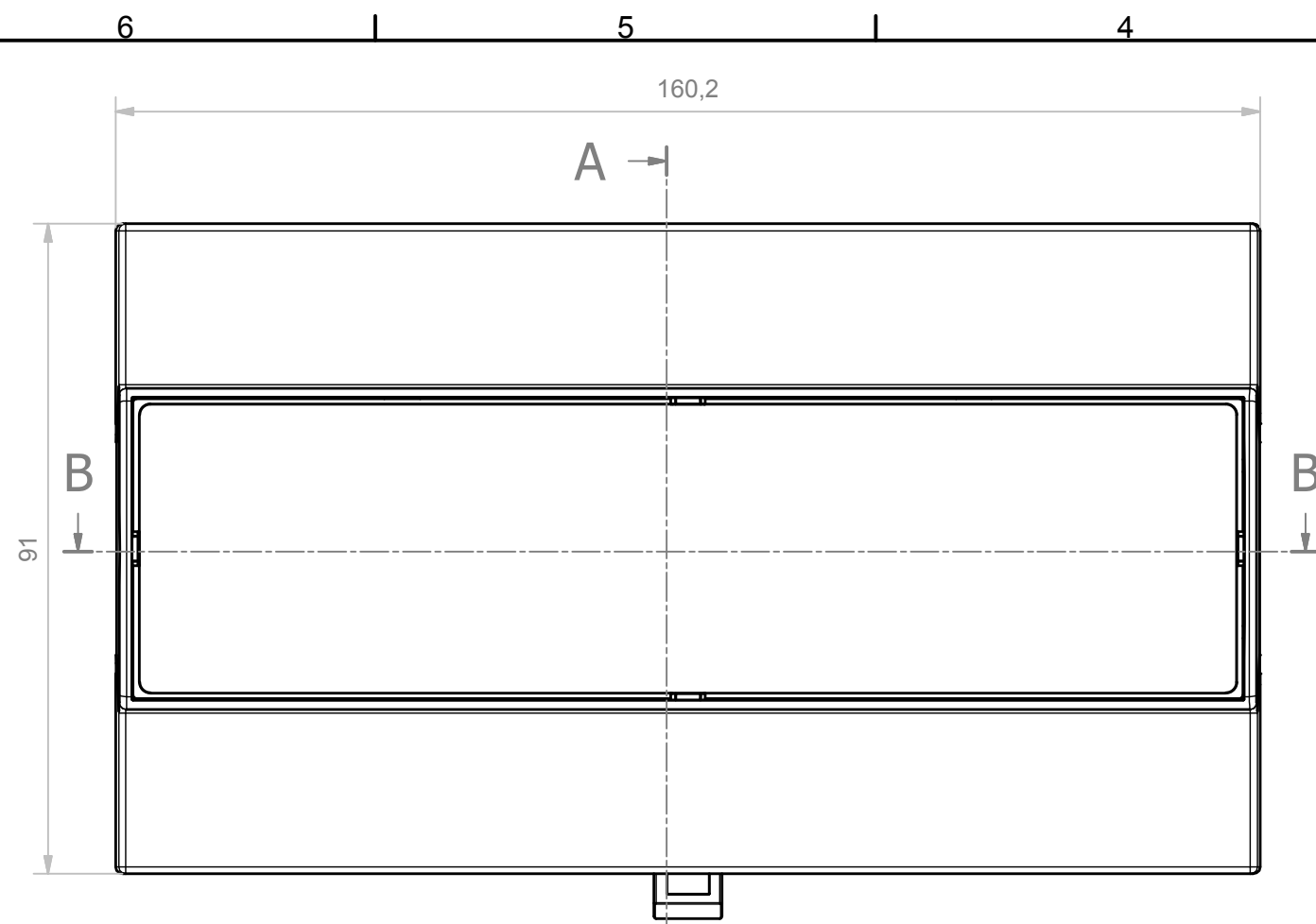
A-A (1:1)
