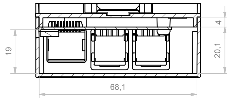
A-A (1:1)
