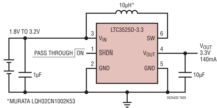
2-Alkaline or NiMH to 3.3V
