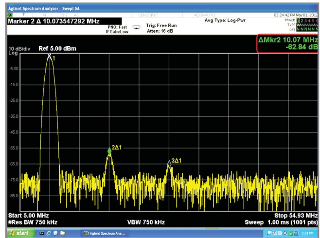
I generatori di forme d'onda Agilent Serie 33500B offrono la più bassa distorsione armonica totale (THD) della categoria.
