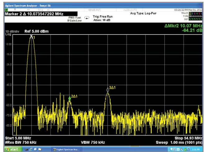
Un tipico generatore DDS presenta un rumore di fondo più elevato e armoniche più grandi.
