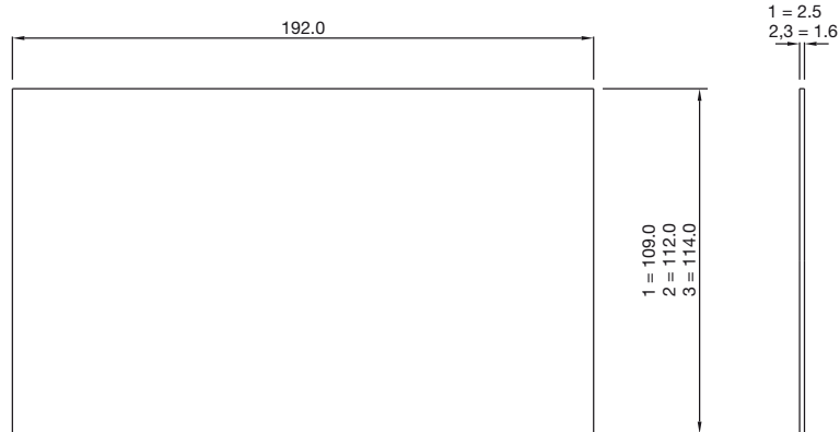
1, 2 & 3 CARD DIMENSIONS DIMENSIONS CARTES 1, 2 & 3
