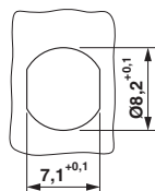
Rysunek wymiarowy
