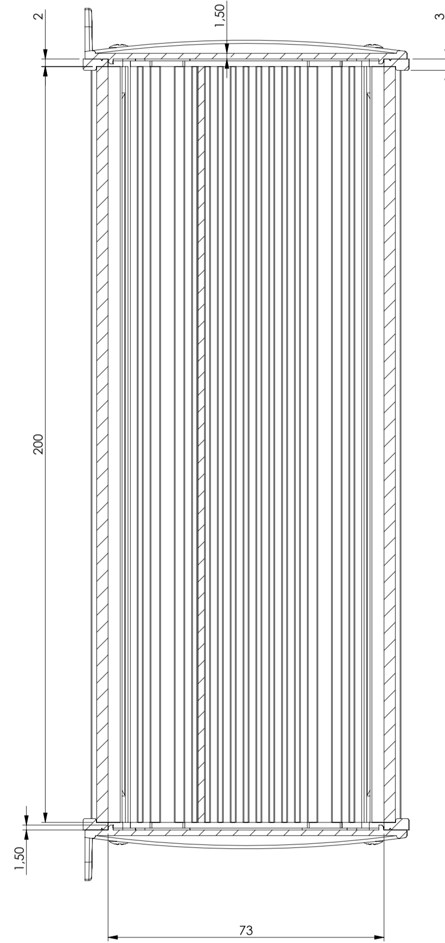
SEZIONE B-B
