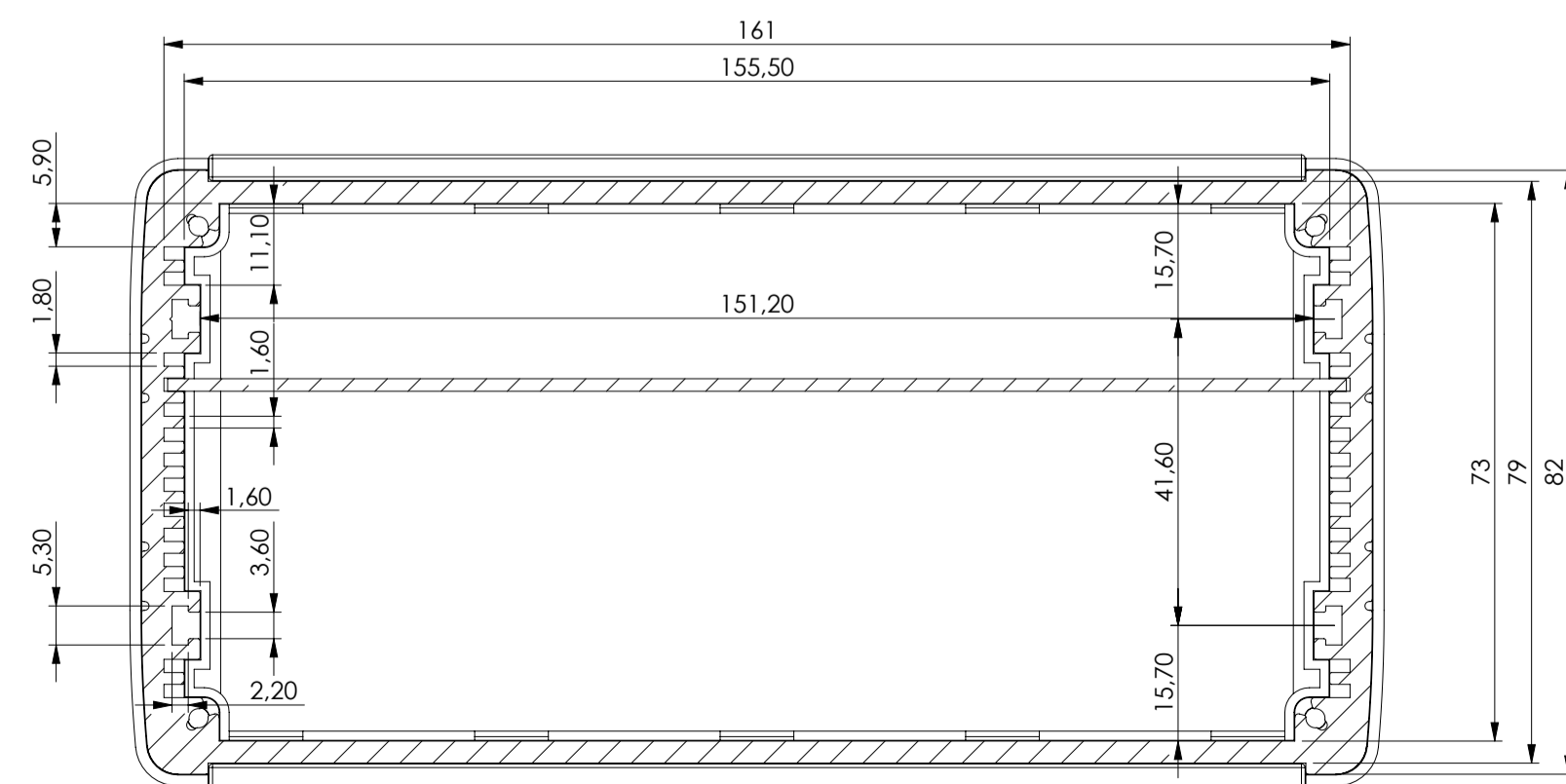
SEZIONE A-A
