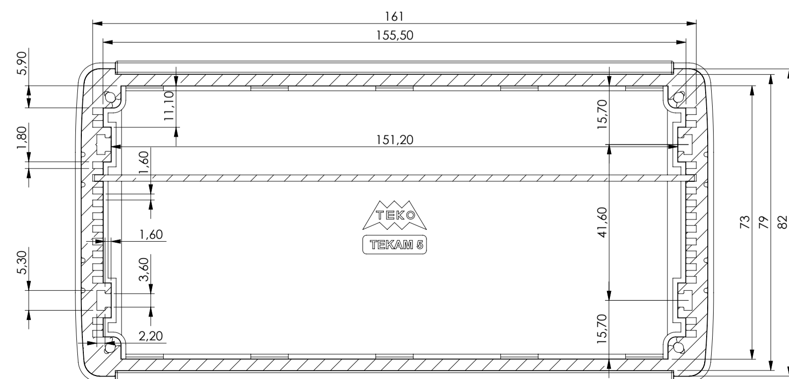
SEZIONE B-B
