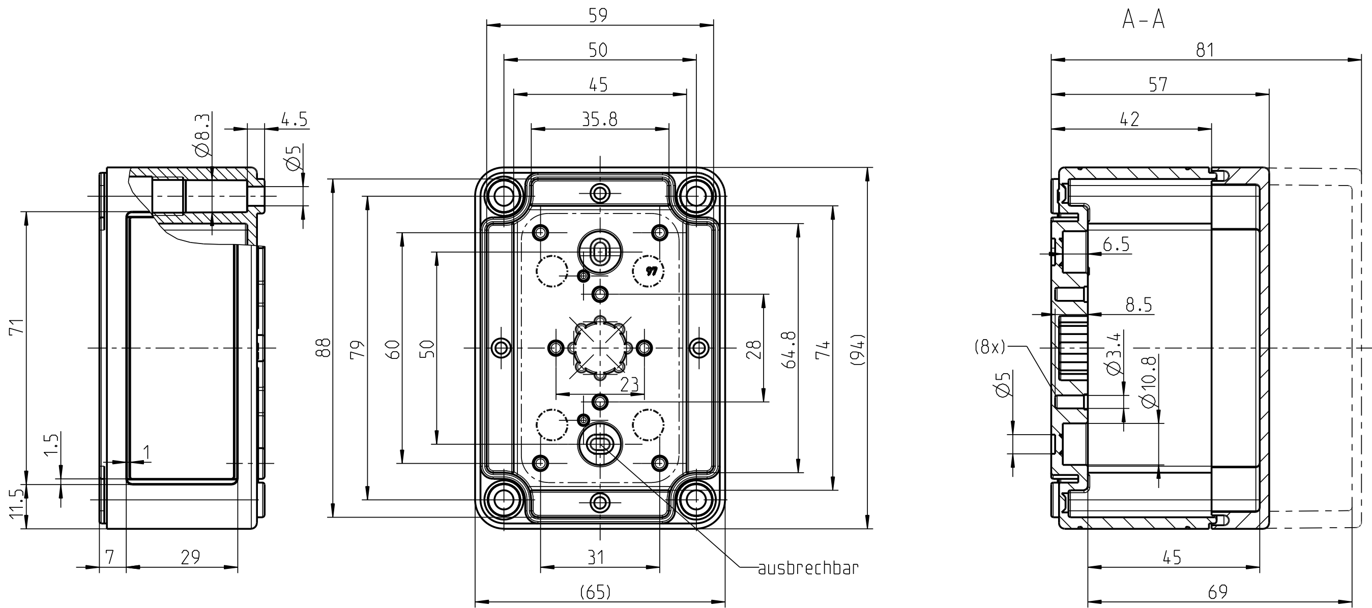
Gehaeuse ohne Vorpraegungen max.moegliche Durchgangsoeffnungen je Kastenseite
