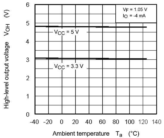
Fig. 12.2.4 V_{OH} - T_a
