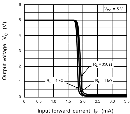
Fig. 13.2.5 V O - I F
