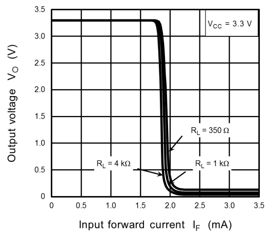
Fig. 13.2.6 V O - I F
