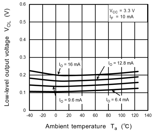
Fig. 13.2.4 V OL - T a
