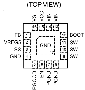
WQFN-16L 3x3
