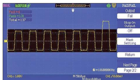
Mode Go-No-Go pour les tests répétitifs selon un gabarit.
