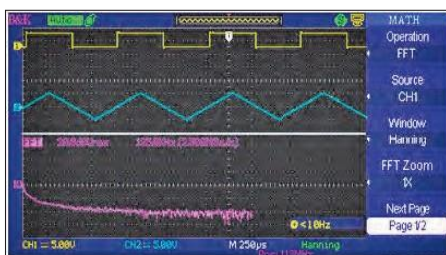
De nombreuses fonctions: FFT avec 4 types de fenêtres.
