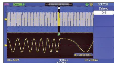
Base de temps retardée, avec zoom sur une partie du signal.
